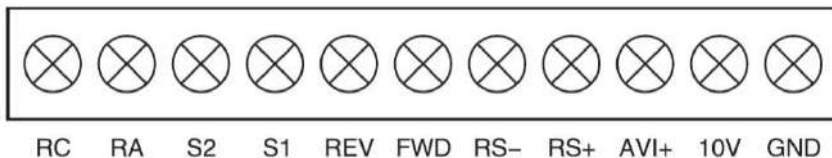
شکل ظاهری ترمینال های فرمان
